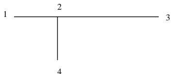
Arbre de longueur minimum
