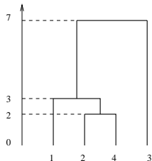
Construction de \delta_{min}
